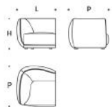
Laterale 97 - versione A Side unit 97 - A version
