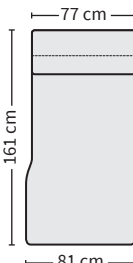
G60L(R)
