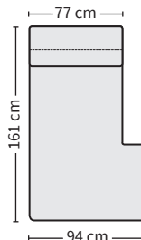
D75R(L)
