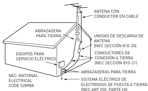
EJEMPLO DE PUESTA A TIERRA DE ANTENA SEGÚN EL CÓDIGO ELÉCTRICO NACIONAL
