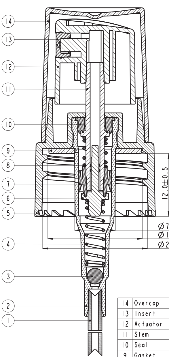
Section A-A
