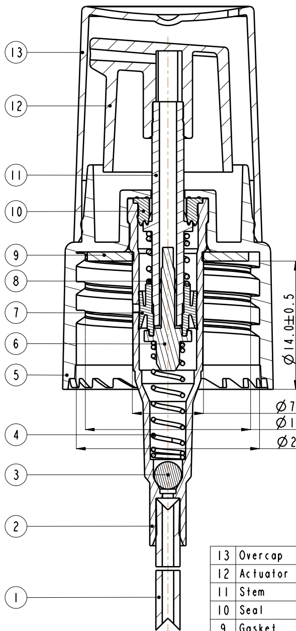
Section A-A
