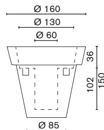
Vas-two container light
