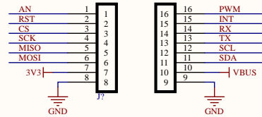
mikroBUS Socket
