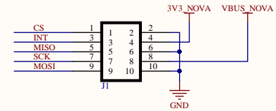
Binho Nova -- SPI
