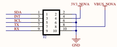
Binho Nova -- I2C
