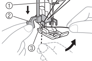
① Supporto dell'ago ② Leva dell'infila ago ③ Guida
