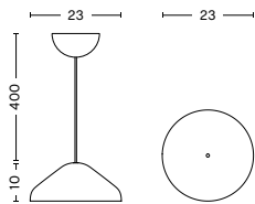
Pao Steel Pendant 230
