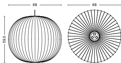
Nelson Ball Bubble Pendant L
