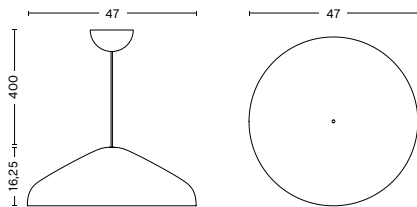
Pao Steel Pendant 470
