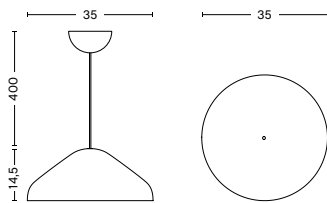
Pao Steel Pendant 350
