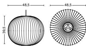
Nelson Ball Bubble Pendant M
