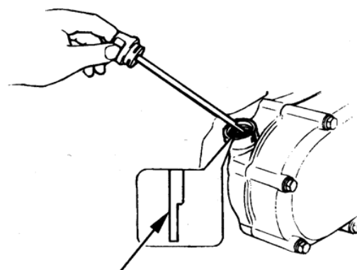
Poziom maksymalny
