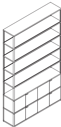
COMBINATION 702 W150 x D34 x H250,5 cm
