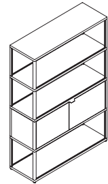
COMBINATION 401 W100 x D34 x H144,6 cm
