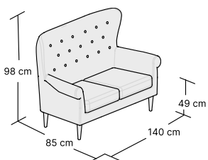
SOFA 2 OSOBOWA W:140 H:98 D:85 cm 1 box
