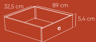
Dimensions intérieures
