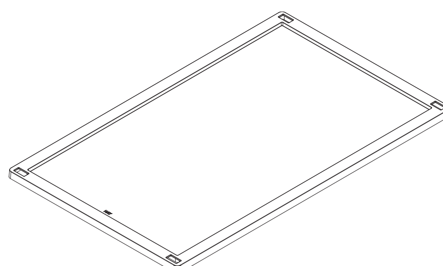
PLASTIC LID X-LARGE W42,5 x L68,5 x H1,5 cm
