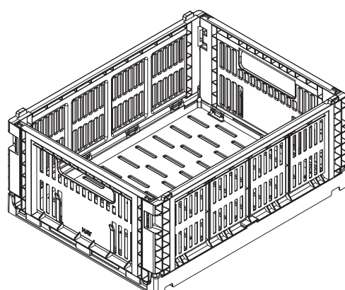
MEDIUM W26,5 x L34,5 x H14 cm
