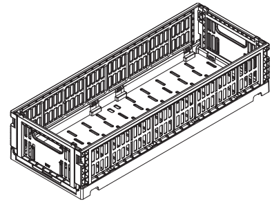
MINI OBLONG W13 x L34,5 x H8 cm
