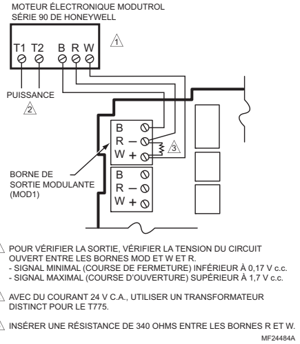
Fig. 19. Raccordement d'un moteur Modutrol série 90.
