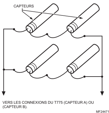
Fig. 3. Raccordement de capteurs en séries parallèles.
