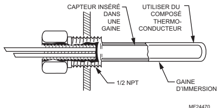
Fig. 2. Capteur inséré dans une gaine d'immersion.
