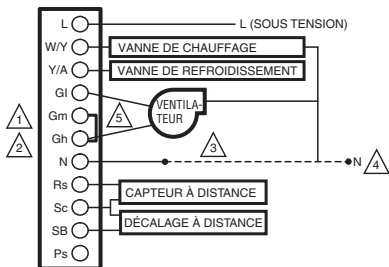
Fig. 12. Schéma de câblage à deux conduits (chauffage ou refroidissement) avec commutation manuelle et chauffage auxiliaire (120/240/277 V c.a. illustré).
