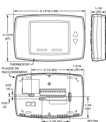
Fig. 1. Dimensions en po (mm).
