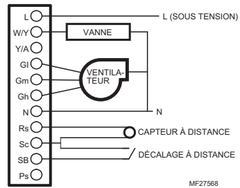
Fig. 9. Schéma de câblage à deux conduits avec commutation manuelle (chauffage ou refroidissement) (120/240/277 V c.a. illustré).
