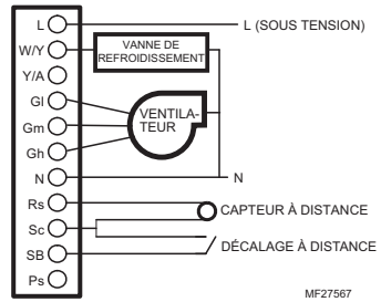
Fig. 8. Schéma de câblage à deux conduits pour refroidissement seulement (120/240/277 V c.a. illustré).
