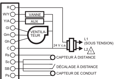
Fig. 18. Schéma de câblage à quatre conduits avec commutation manuelle/automatique (chauffage et refroidissement) (24 V c.a. illustré).
