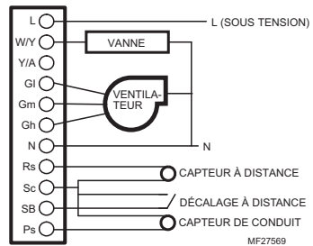
Fig. 10. Schéma de câblage à deux conduits (chauffage ou refroidissement) avec commutation automatique (120/240/277 V c.a. illustré).
