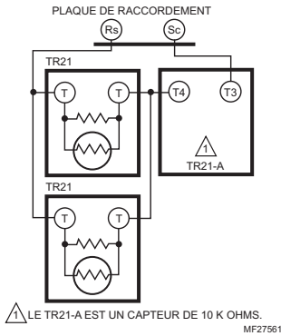
Fig. 6. Câblage de deux capteurs TR21 (20 K ohms) et d'un capteur TR21-A (10 K ohms) pour fournir un réseau de moyenne de température.
