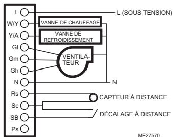
Fig. 11. Schéma de câblage à quatre conduits (chauffage ou refroidissement) avec commutation manuelle/automatique (120/240/277 V c.a. illustré).
