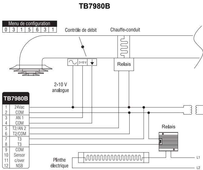
FIGURE 1 : Contrôle de débit avec chauffe-conduit et chauffage auxiliaire par plinthe électrique
