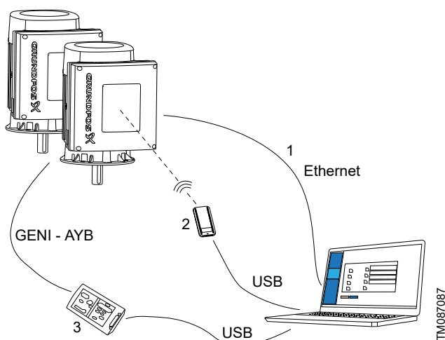
Grundfos GO Link setup
