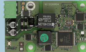
CIM module
