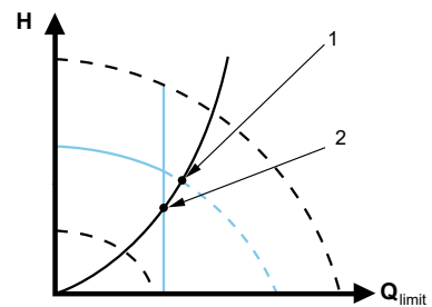
Courbe constante avec FLOW_{LIMIT}
