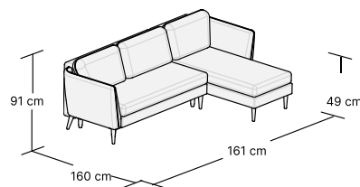
NAROŻNIK Z SZEZLONGIEM I FUNKCJĄ SPANIA UNIWERSALNY LEWY W:250 H:91 D:160 cm 2 boxes BED: 210x140 cm
