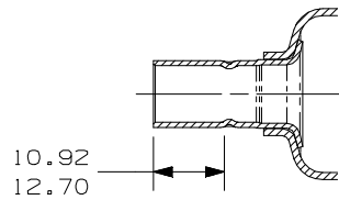
CORTE A-A ESCALA 1:1
