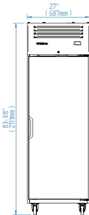
ELEVATION
