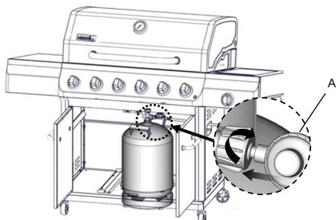
A. Gastryksregulator/slangesamling
